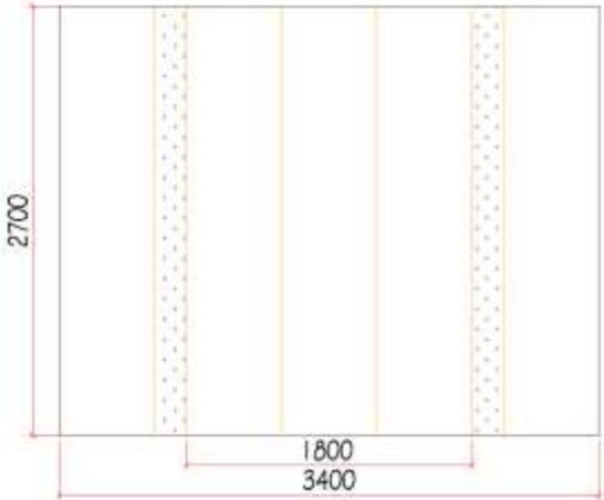
Minisize : 3400mm
