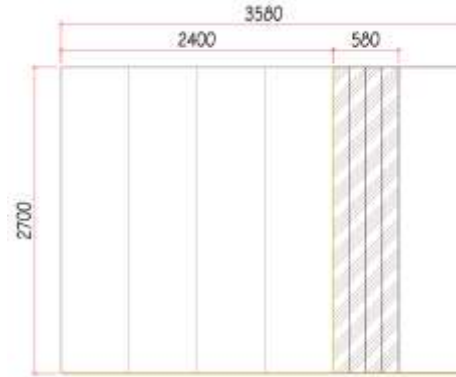
Minisize : 3580mm
