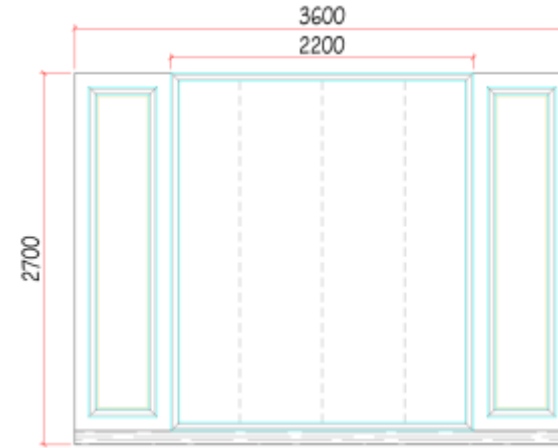
Minisize : 3600mm
